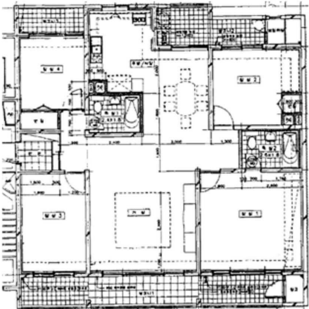
내부구조도
