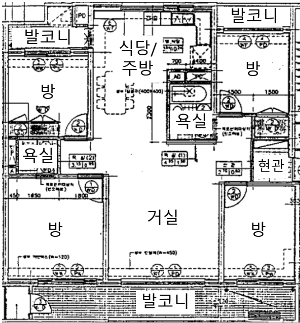
[내부구조도]
